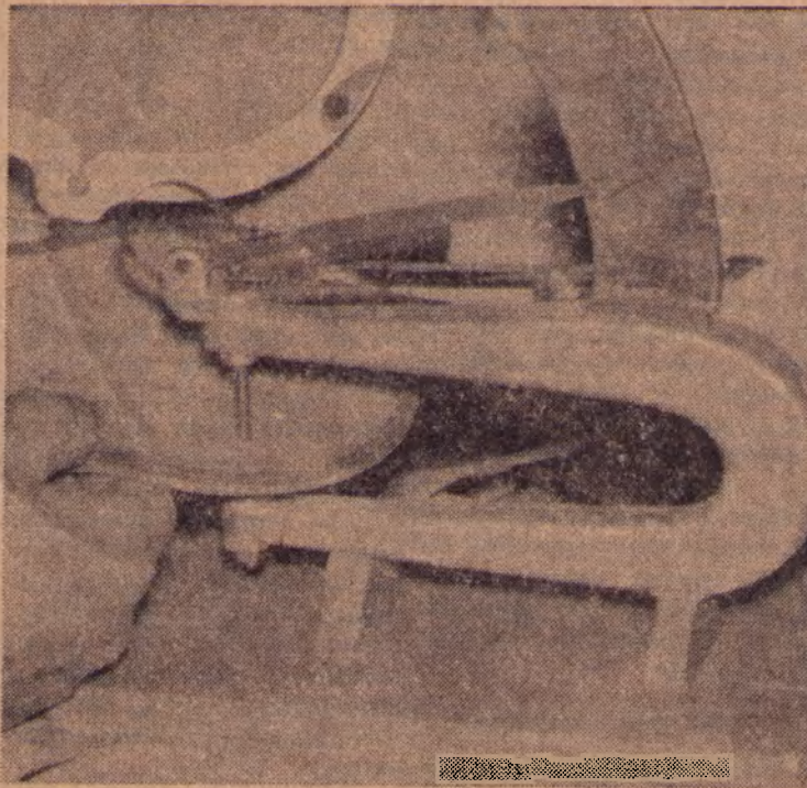
Med det här mätverktyget — som är hemmagjort — mäts stockleken på botten och lock i fiolen. Det är mycket viktigt att måtten är de riktiga.
